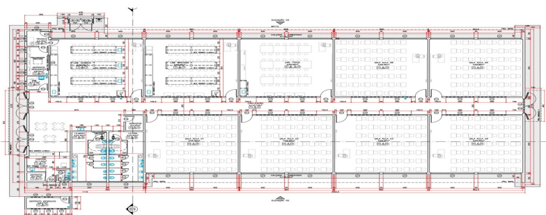
Figura 4: Bloco Didático
